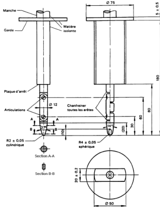
Figure n°1 : Calibre d'essai B (doigt d'épreuve articulé)
